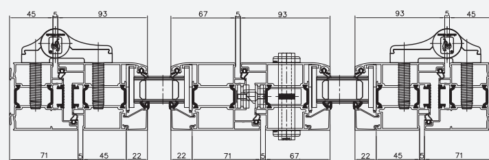
Coupe horizontale
